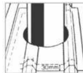
3. Rajzolja fel a Dektite vízzáró gumiharang kontúrját a tetőn. Távollítsa el a gumiharangot és jelöljön fel 30 mm-es rátartást.
