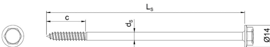
Bild 2: Dübeltyp Kragenkopf mit Bund (KB)
